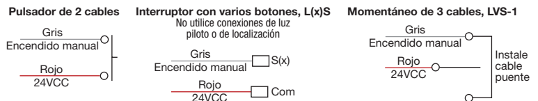
Cableado de la opción de interruptor momentáneo de bajo voltaje
