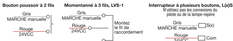
Câblage de l'interrupteur momentané basse tension facultatif
